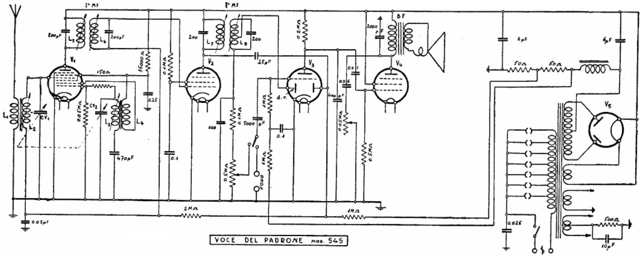
Fig. 29. - Schema di ricevitore supereterodina di tipo commerciale.
